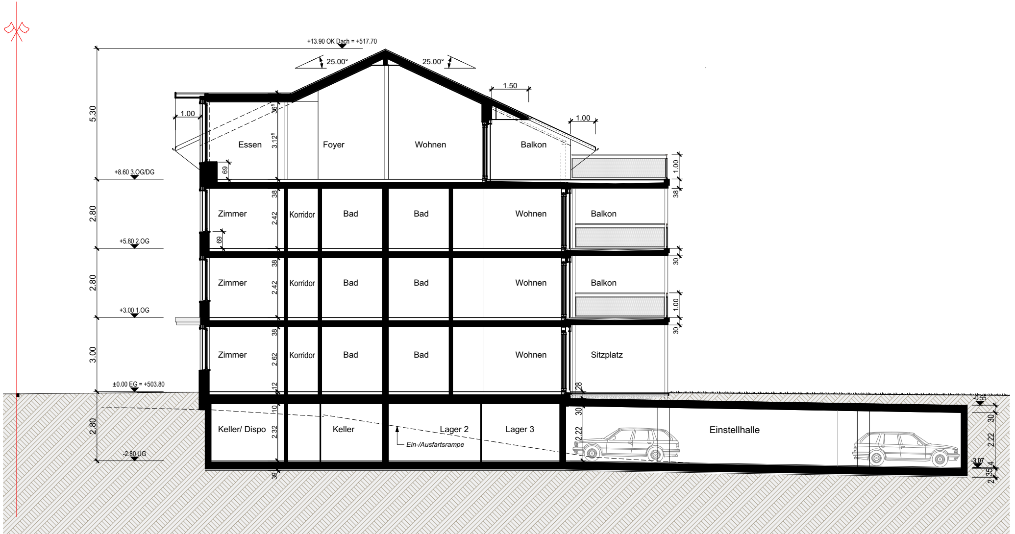
Querschnitt
