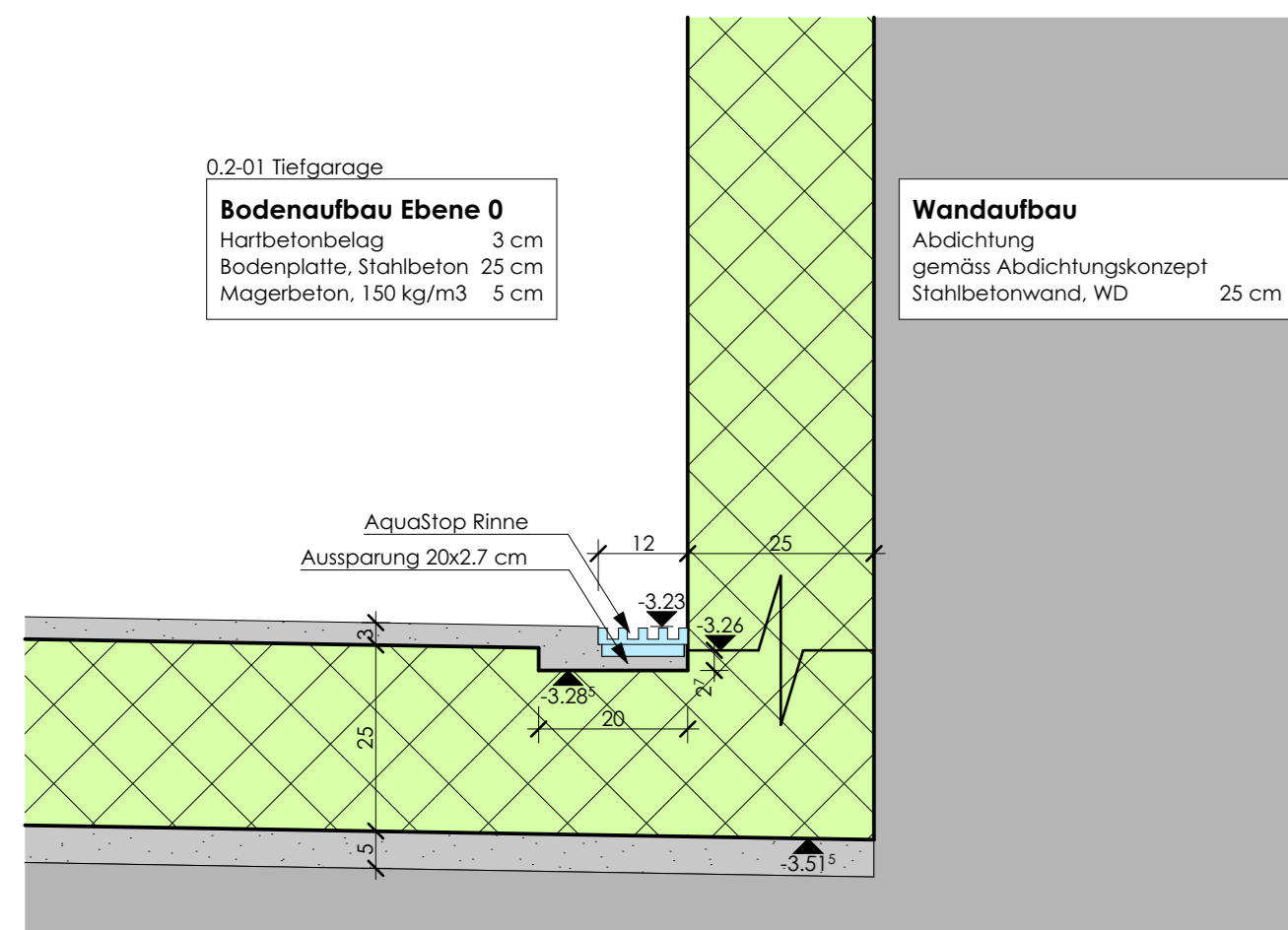
D1 Entwässerung Einstellhalle MST 1:10
